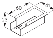
SG 11238 Nutmaske
