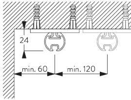
Träger SG 6124
