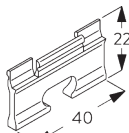
SG 5118 Klammer
