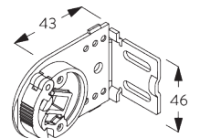
SG 10990 Träger, fensterseitig abrollend
