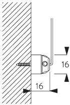
Einzelssystem
