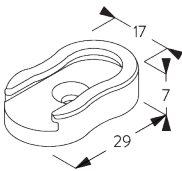
SG 10673 Doppelhalter kurz Seitenführung kurz
