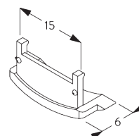
SG 10684 Trägerabdeckung
