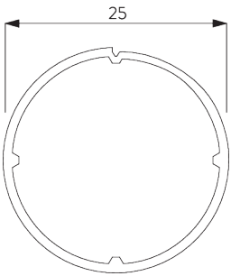
SG 10533 Rohr ø 25 mm
