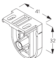
SG 10680 Träger Lagerseite
